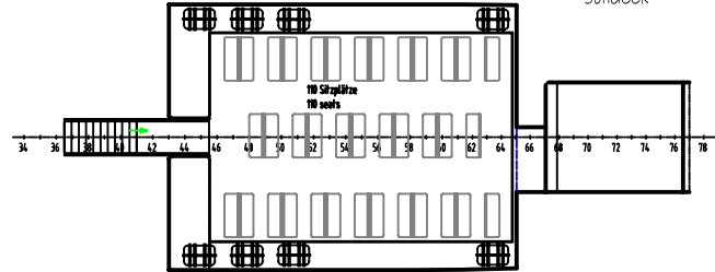
Sonnendeck sundeck
